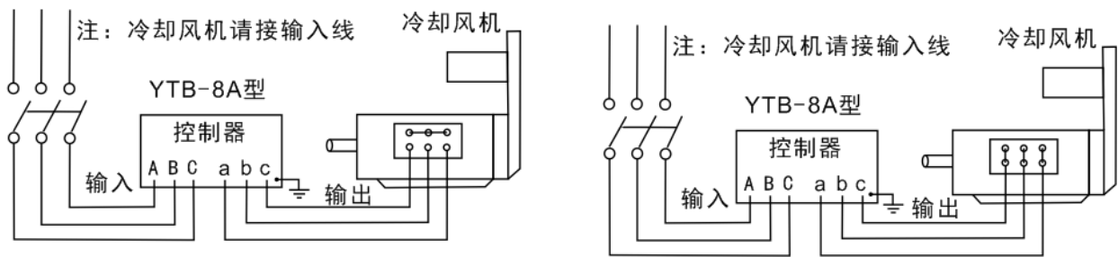
YTB-8A 型力矩控制仪接入 Y 型、 \Delta 型力矩电机接线图
